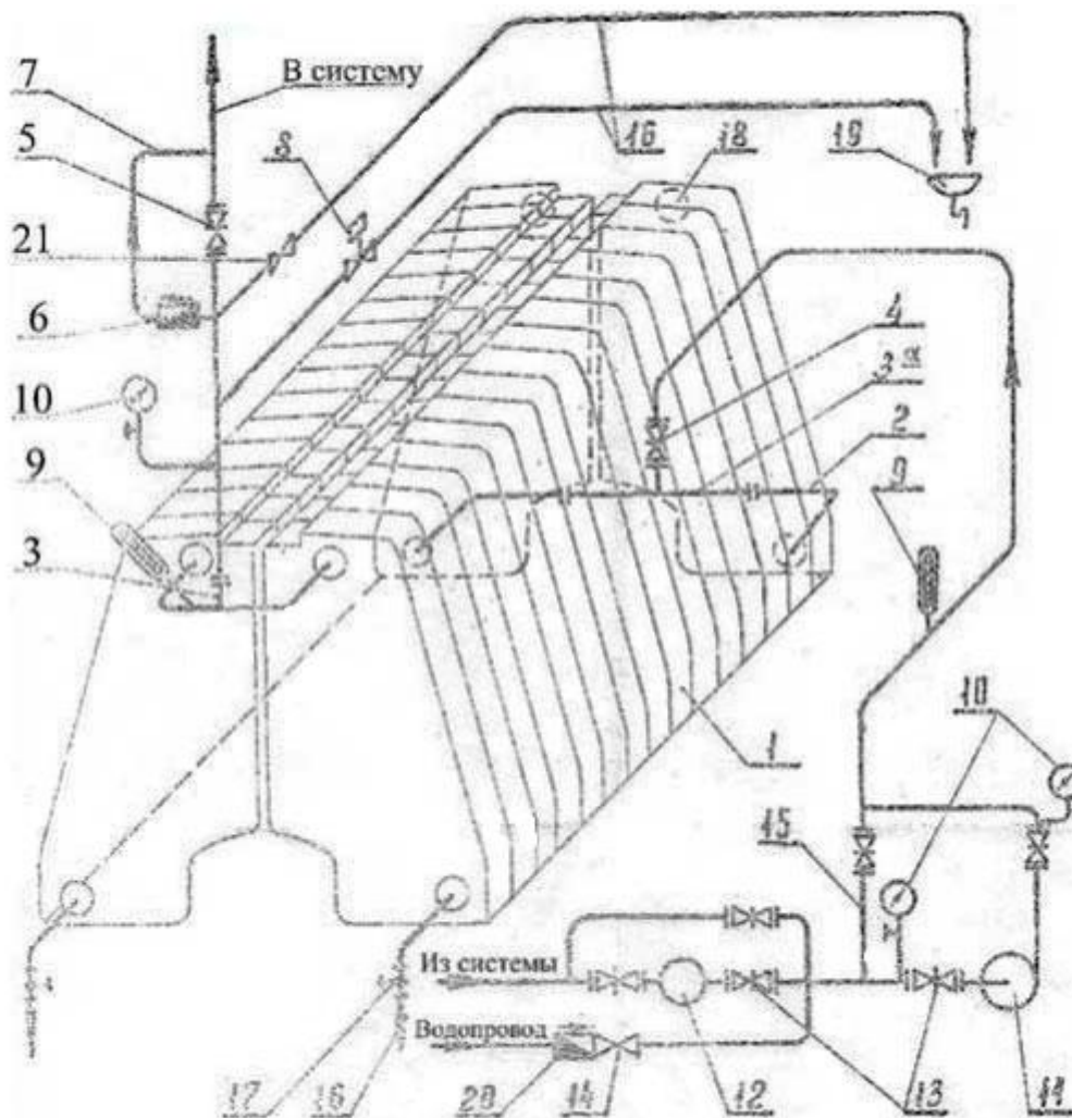
Схема котла Универсал 6
