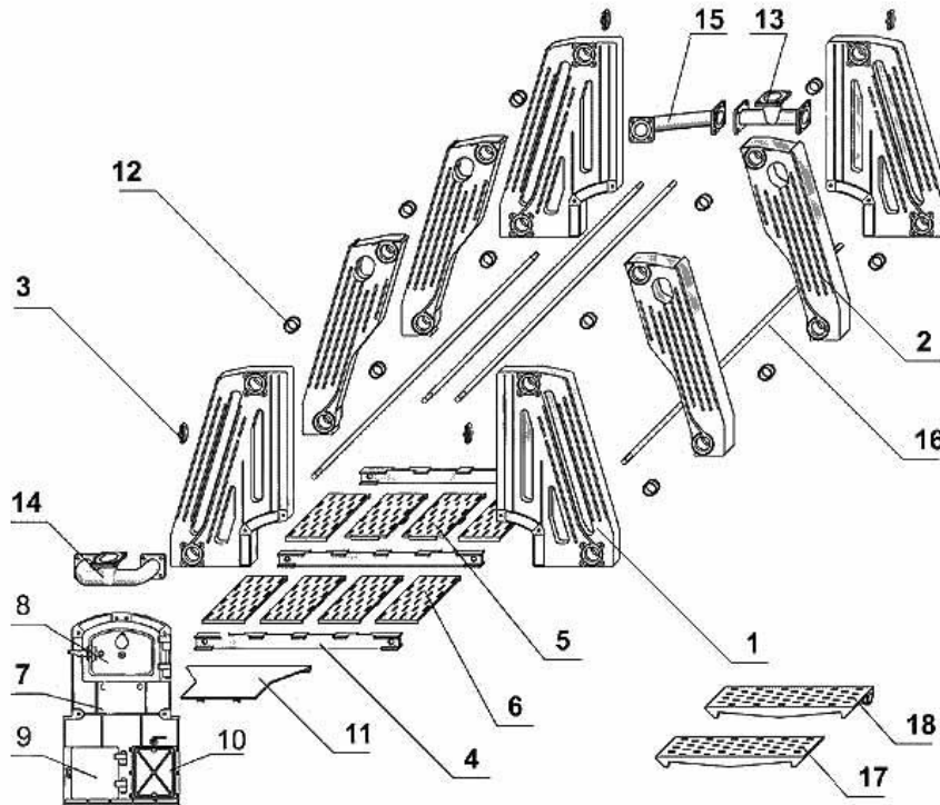
Монтажная схема котла Универсал 6
